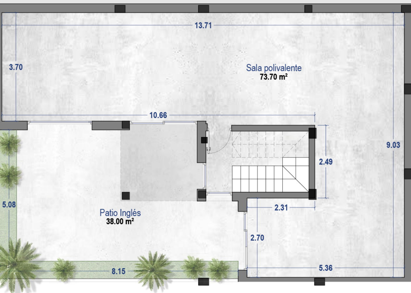
PLANTA SÓTANO
