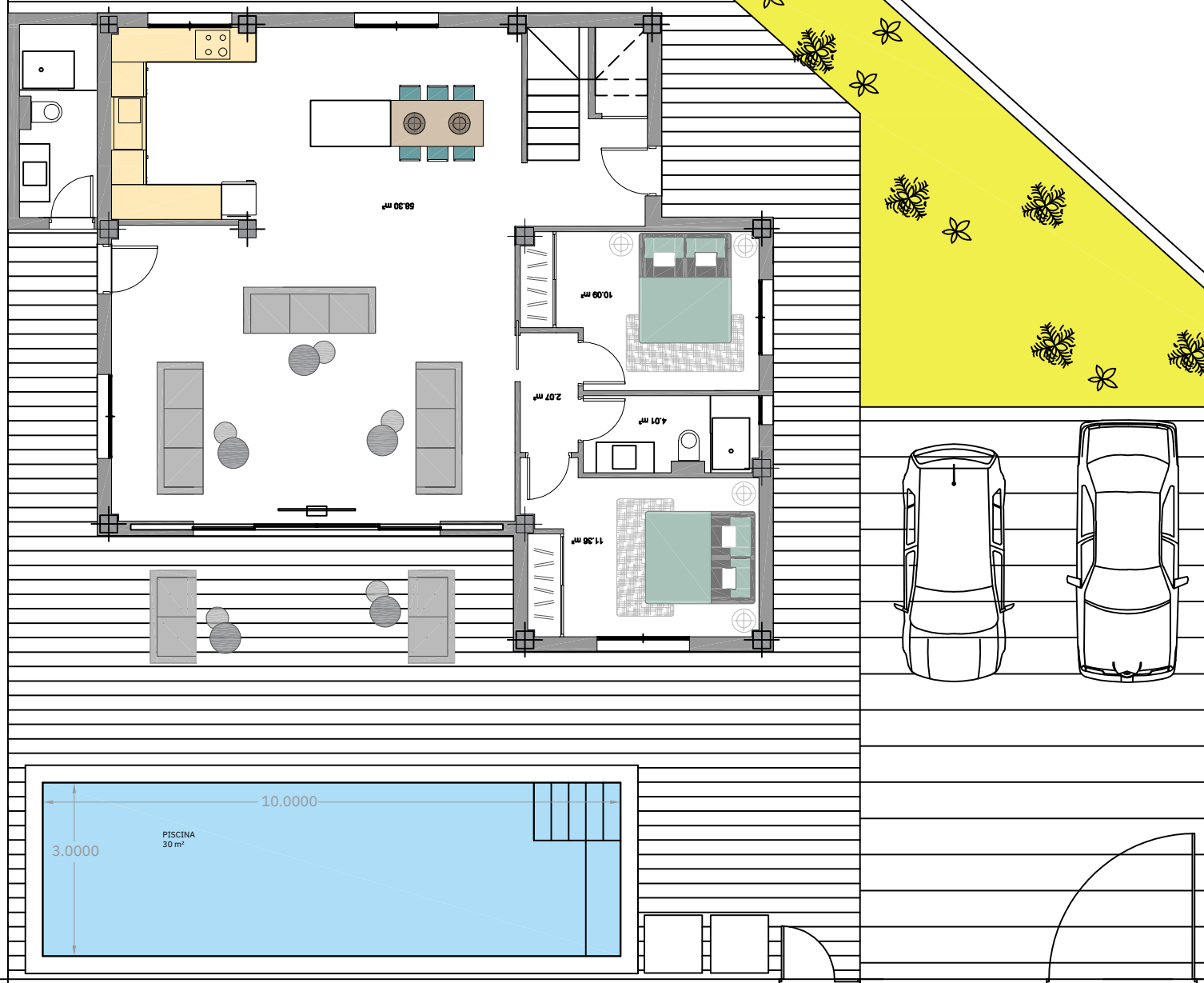
PLANTA BAJA
