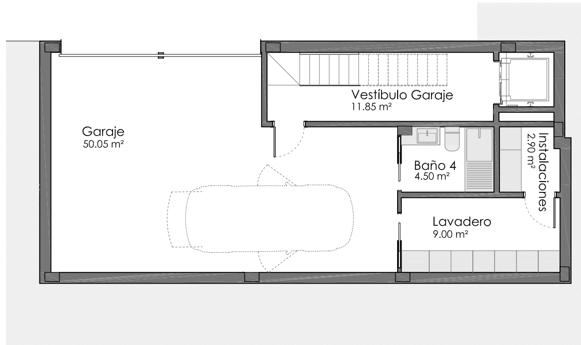
SEMISÓTANO. NIVEL -1
