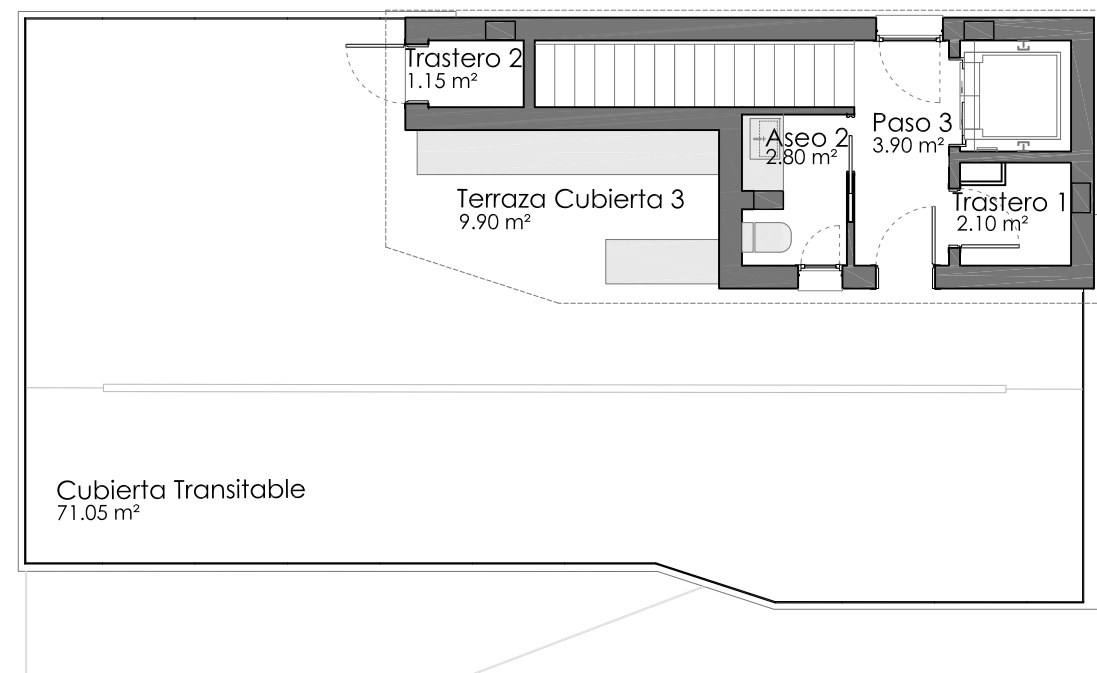
TORREÓN. NIVEL 3
