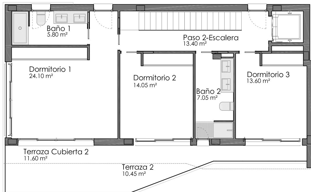
PLANTA 1. NIVEL 2
