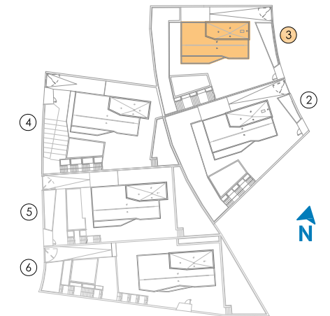
SEMISÓTANO. NIVEL -1
